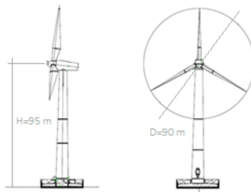
Figura 8 Schema aerogeneratore
